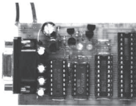
Рис.1. Програматор «EXTRA-PC»
